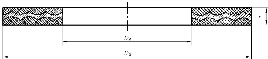
图 1 基本型
