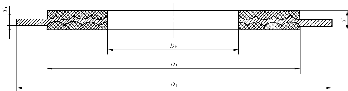
图 2 带定位环型
