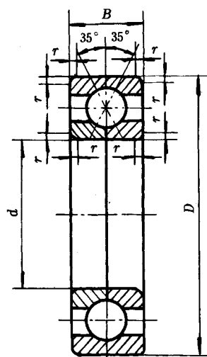
图 2 四点接触球轴承 QJ 型
