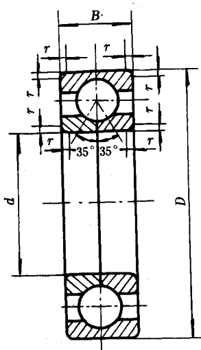
图 1 三点接触球轴承 QJS 型
