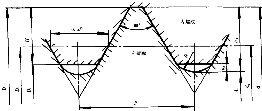
设计牙型的尺寸
