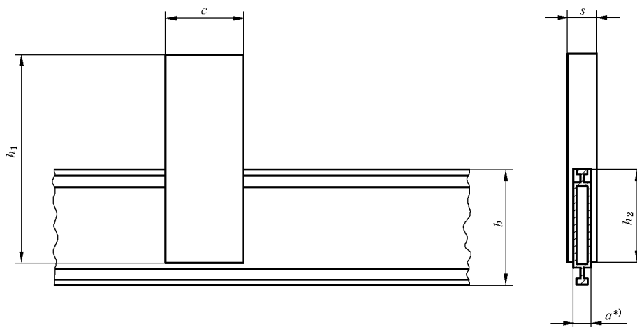
图1 综框导板
