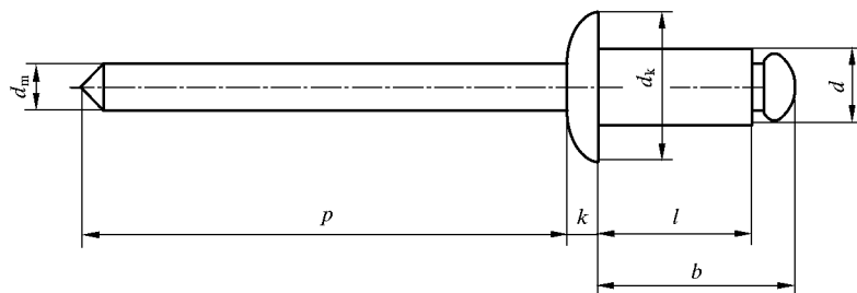
图 1 铆钉尺寸
