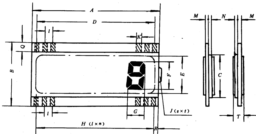
图1 尺寸标注
