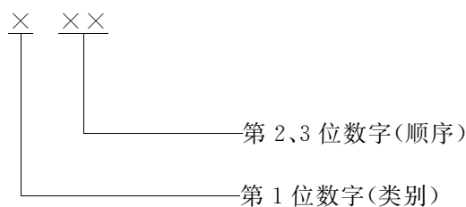
图 1 代码结构图
