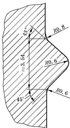
图 1 铣刀轮廓
