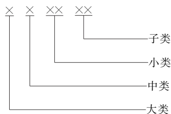
图 1 代码结构图
