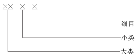
图 1 代码结构图
