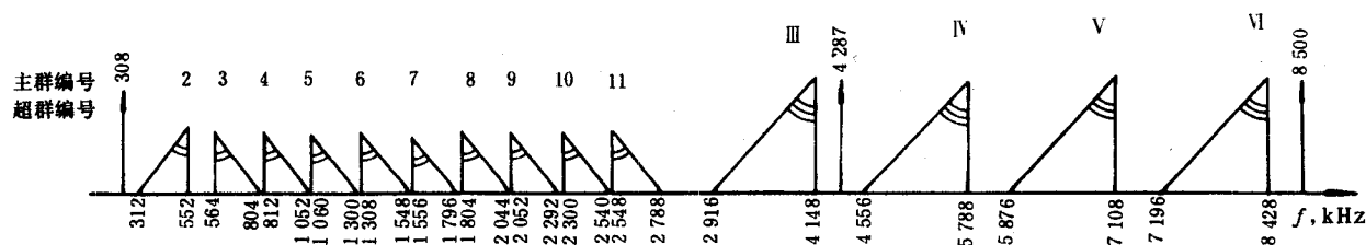
图 1 线路频谱
