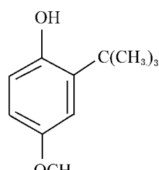
3-叔丁基-4-羟基茴香醚
