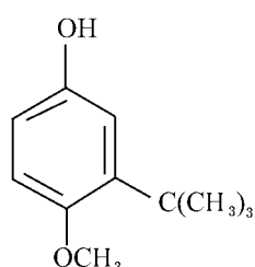
2-叔丁基-4-羟基茴香醚
