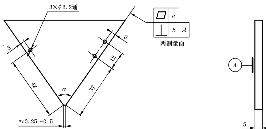
图 1 I 型角度量块的型式示意图
