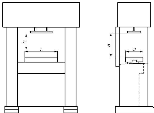
图 1 电解去毛刺机床
