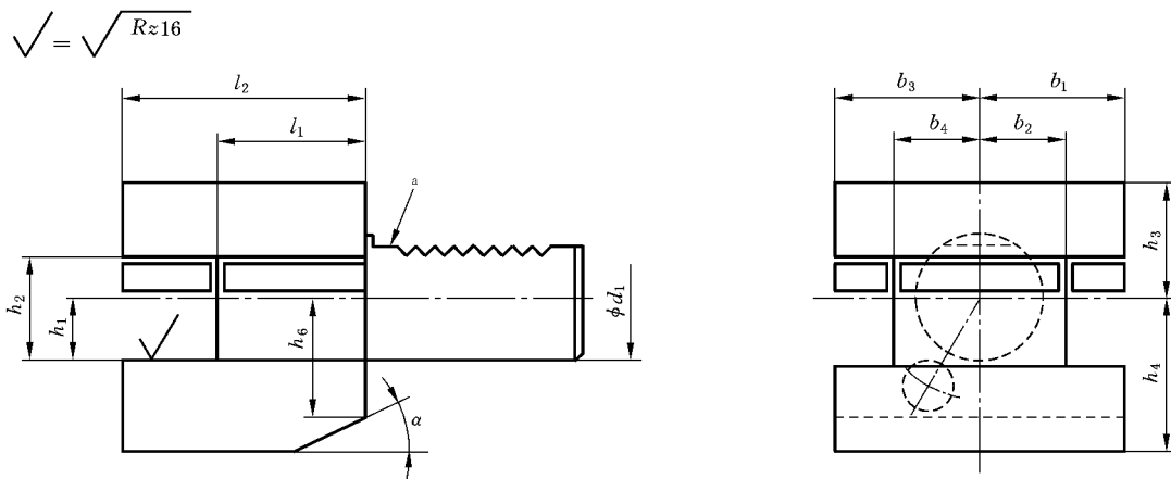
图 1 D1 型刀夹
