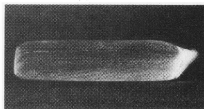
图 2 分层裂纹(侧向截面)1.5×
