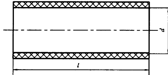
图1 圆柱形筒管
