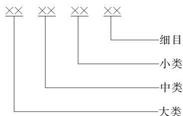
图 1 代码结构图
