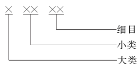
图 1 代码结构图
