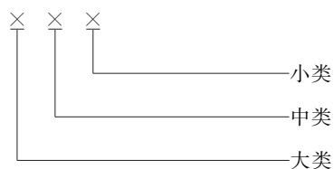
图 1 代码结构图
