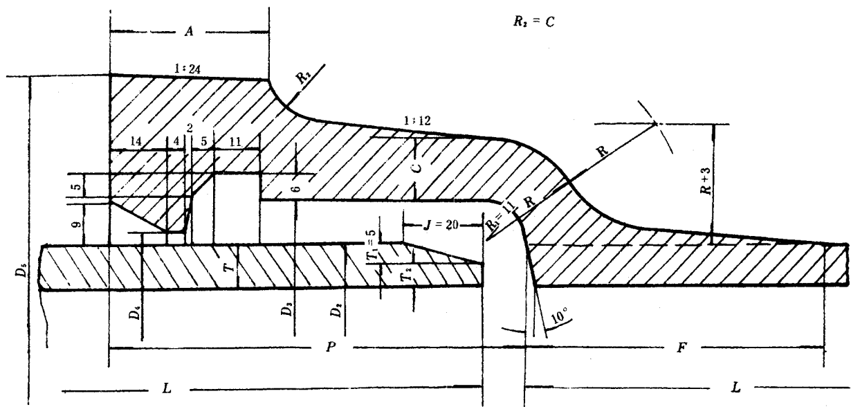
图 1 梯唇型橡胶圈接口铸铁管
