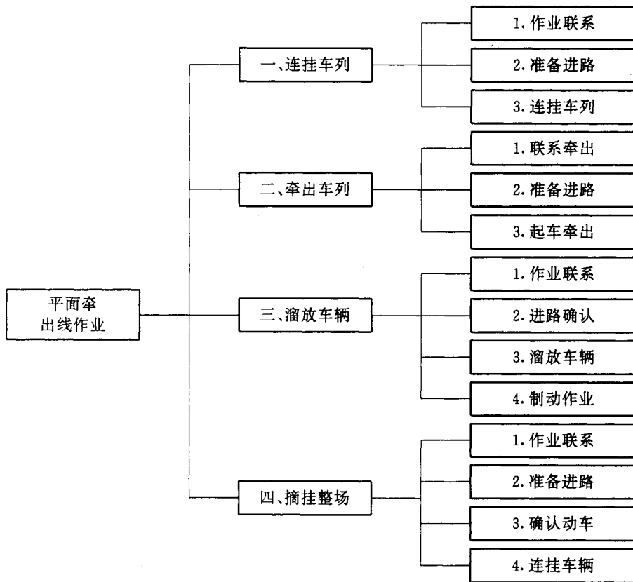
图1 铁路调车平面牵出线作业程序图
