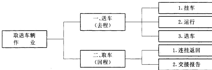
图 1 铁路调车取送车辆作业程序图
