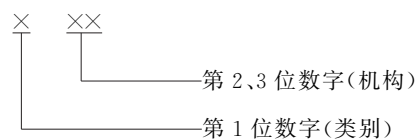
图 1 代码结构图
