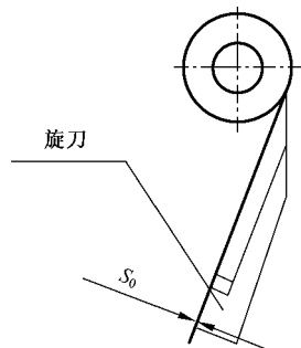
图1 刀门间隙示意图
