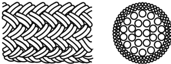
图 1 聚酯复丝绳索双层编织结构
