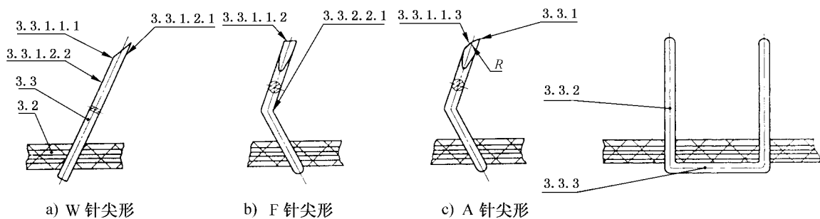
图 1 弹性针布
