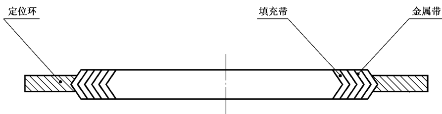
图 3 带定位环型
