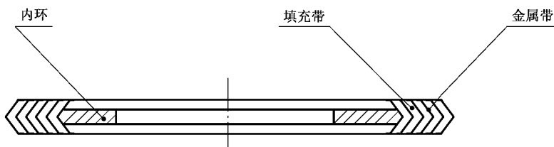
图 2 带内环型
