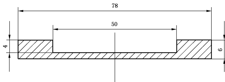
图 1 盛样槽剖面图
