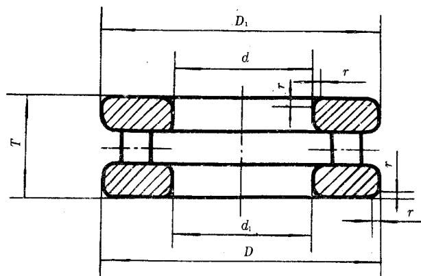
推力圆柱滚子轴承 80000 型
