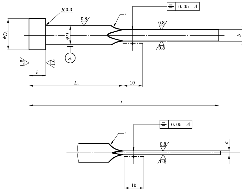
图 1 扁推杆
