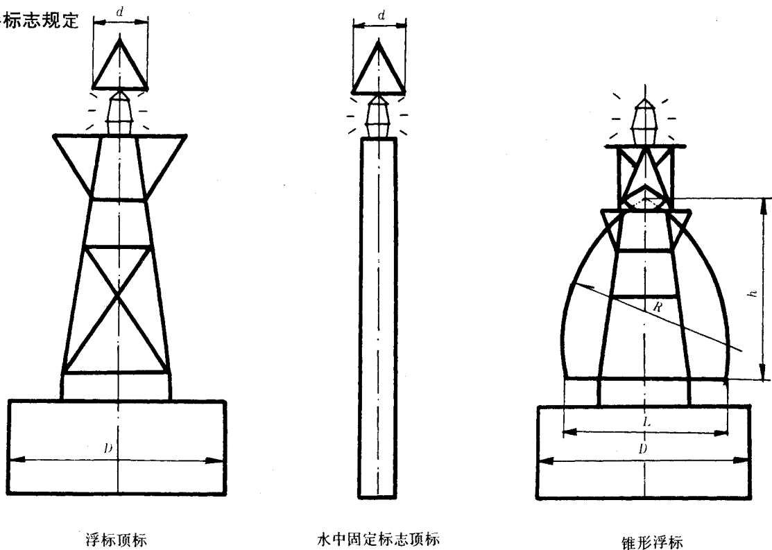
图1 锥形标志
