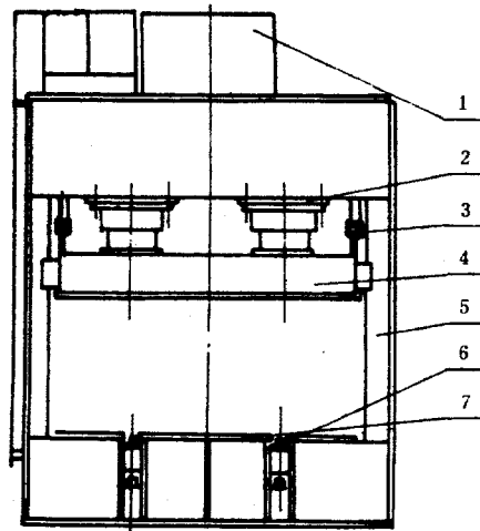
1—液压系统；2—主油缸；3—提升缸；4—活动横梁； 5—机架；6—输送机构；7—固定横梁
