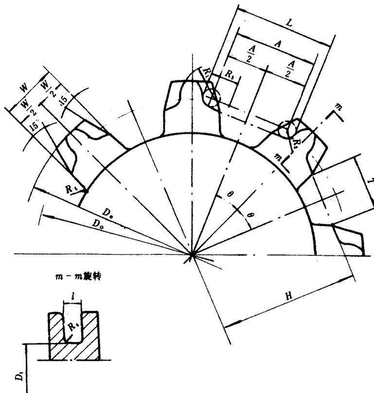
图 1 链轮型式和尺寸
