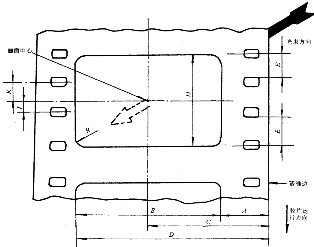
图1 35mm电影摄影底片的画面面积
