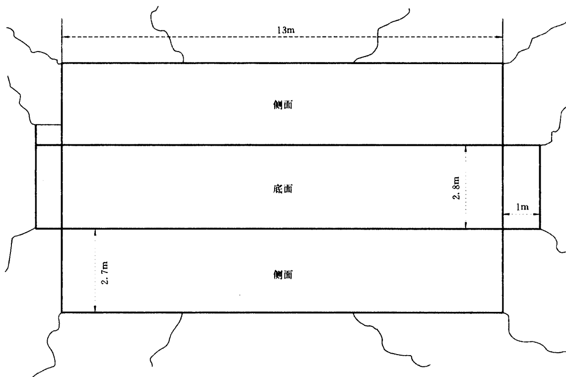
图 1 大袋规格示意图
