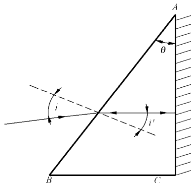
图 1 自准直法测量原理图
