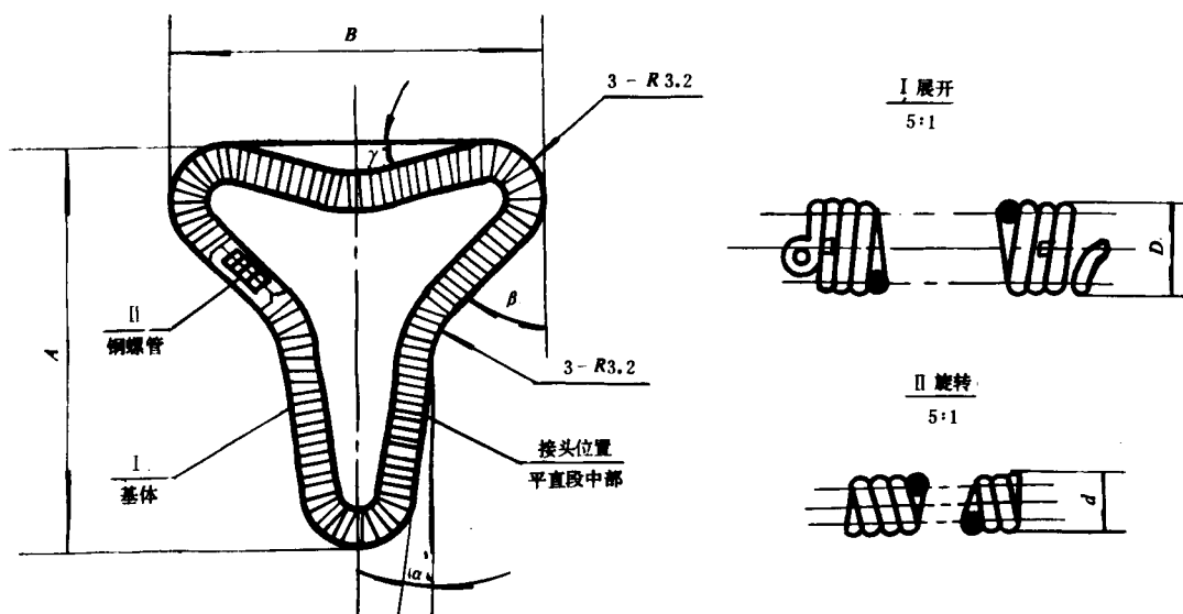
图1 含铜宫内节育器
