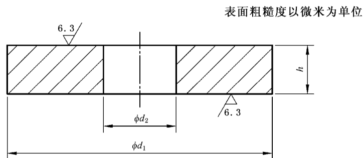
图1 弹簧环
