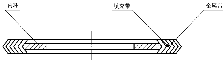
图 2 带内环型
