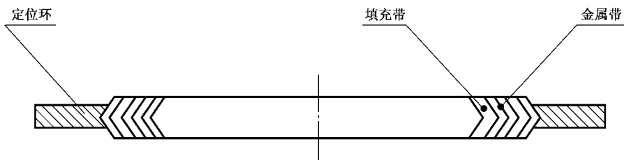
图 3 带定位环型
