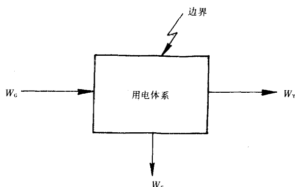
图1 电能平衡的基本模型图
