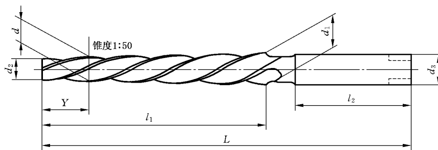
图 1 直柄机用 1 : 50 锥度销子铰刀型式
