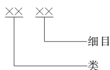
图 1 代码结构图
